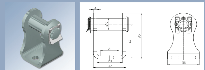
EEL900BA60-3KS (côté tige) Charge max : 5000N, Matière : acier zingué
