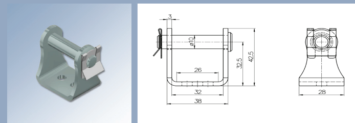
EEL900BA50-2MS (côté moteur) Charge max : 4500N, Matière : acier zingué
