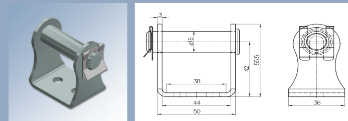
EEL900BA60-3MS (côté moteur) Charge max : 5000N, Matière : acier zingué
