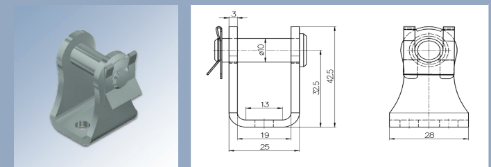
EEL900BA50-2KS (côté tige) Charge max : 4500N, Matière : acier zingué
