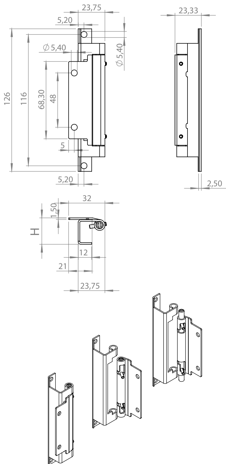
120° - Hinge
