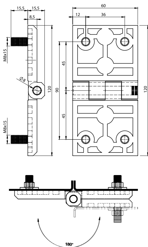
3014, 3022 - 180° Hinge
