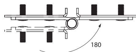
3114, 3113, 3093 - 180° Hinge
